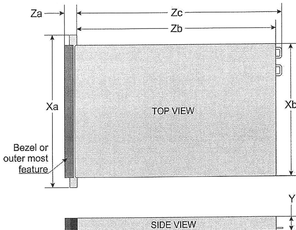
Figura 1. Dimensiunile șasiului PowerEdge R450
